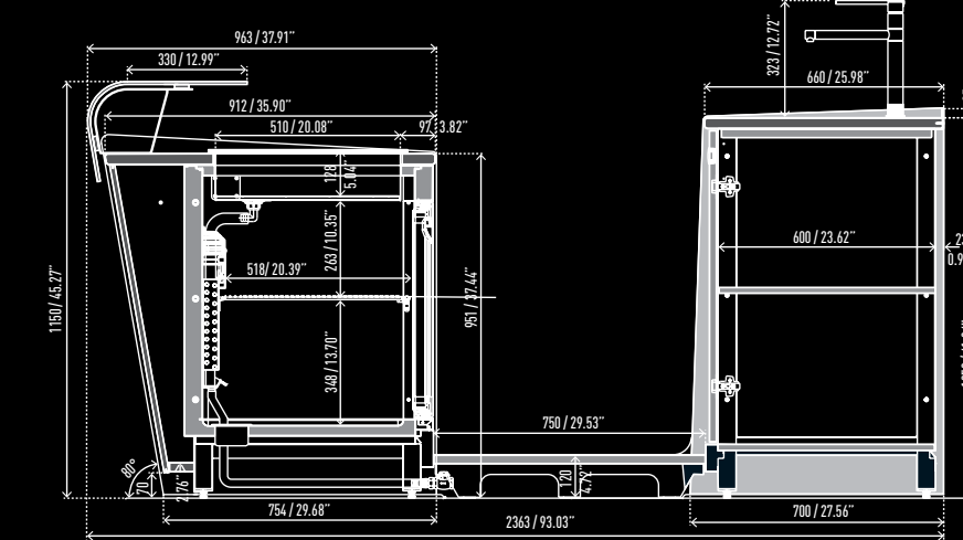
START UP H 951 BC / H 1150 con bancalino in vetro - with glass countertop - avec plan de comptoir en verre - mit Ablagefläche aus Glas - con encimera de vidrio
