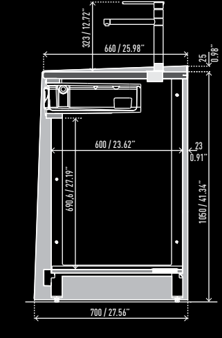
VANO LAVELLO Sink - Evier - Spülbecken - Fregadero
