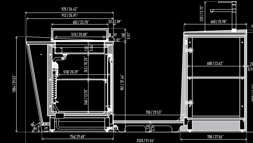
START UP H 951 PL con copertura in plexiglas - with Plexiglas cover - avec couvercle en plexiglas - mit Plexiglasabdeckung - con cubierta de plexiglas
