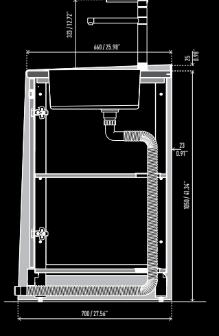
VANO LAVA TAZZE Glass washer - Lave Tasses - Tassenspüler - Lavatazas
